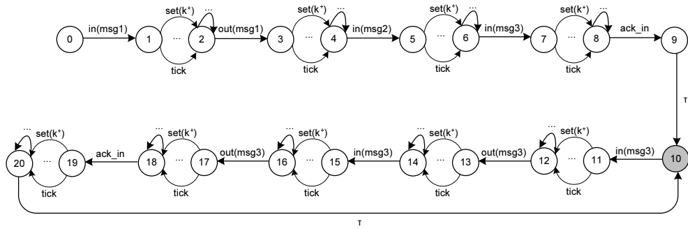
Figure 7.12: Violation pattern for PAR
